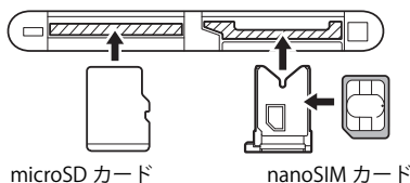
microSD カード
